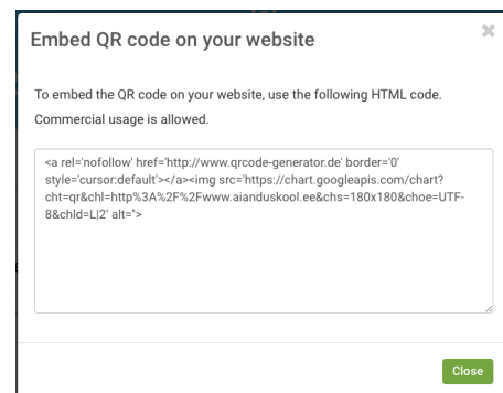
Joonis 6. QR-koodi embeedimise ehk vistutamise html kood
